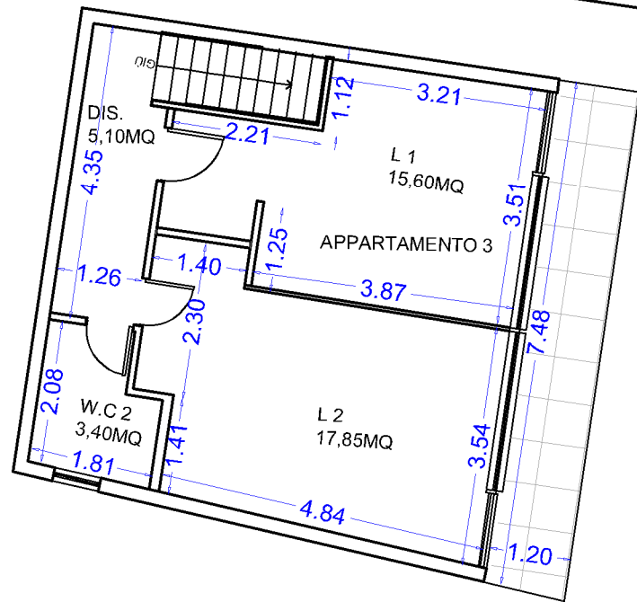
CORPO D2 (LIVELLO PRIMO)
